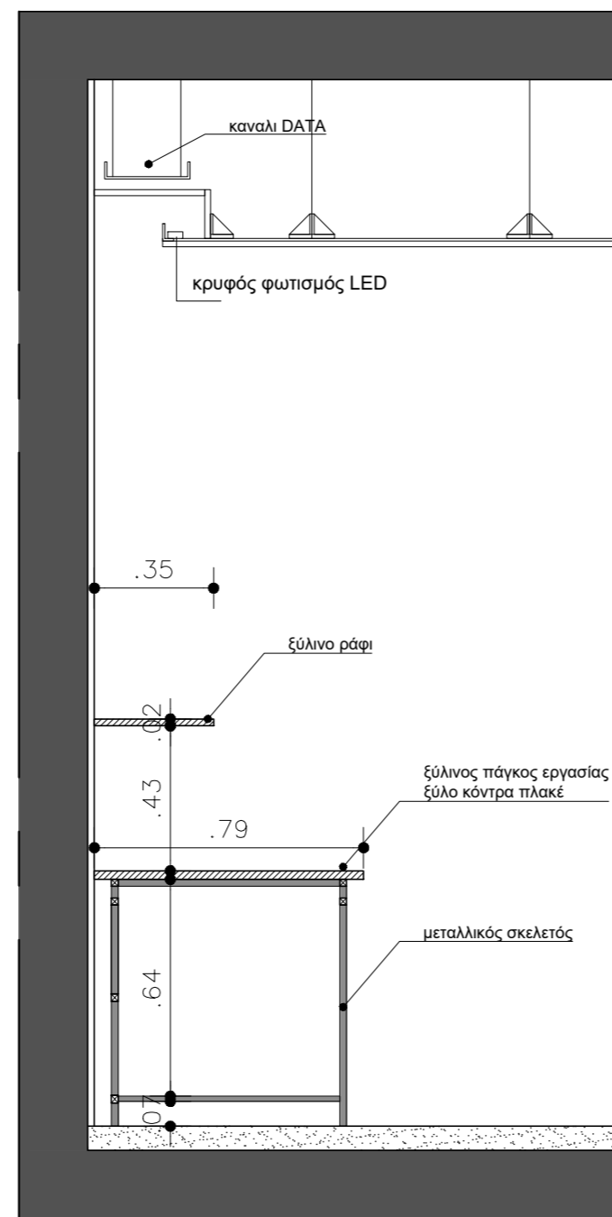
ΛΕΠΤΟΜΕΡΕΙΑ ΚΡΥΦΟΥ ΦΩΤΙΣΜΟΥ
