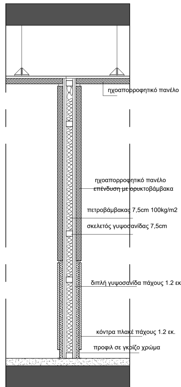
ΛΕΠΤΟΜΕΡΕΙΑ ΚΑΤΑΣΚΕΥΗΣ ΔΙΑΧΩΡΙΣΤΙΚΟΥ ΠΕΡΑΣΜΑΤΟΣ
